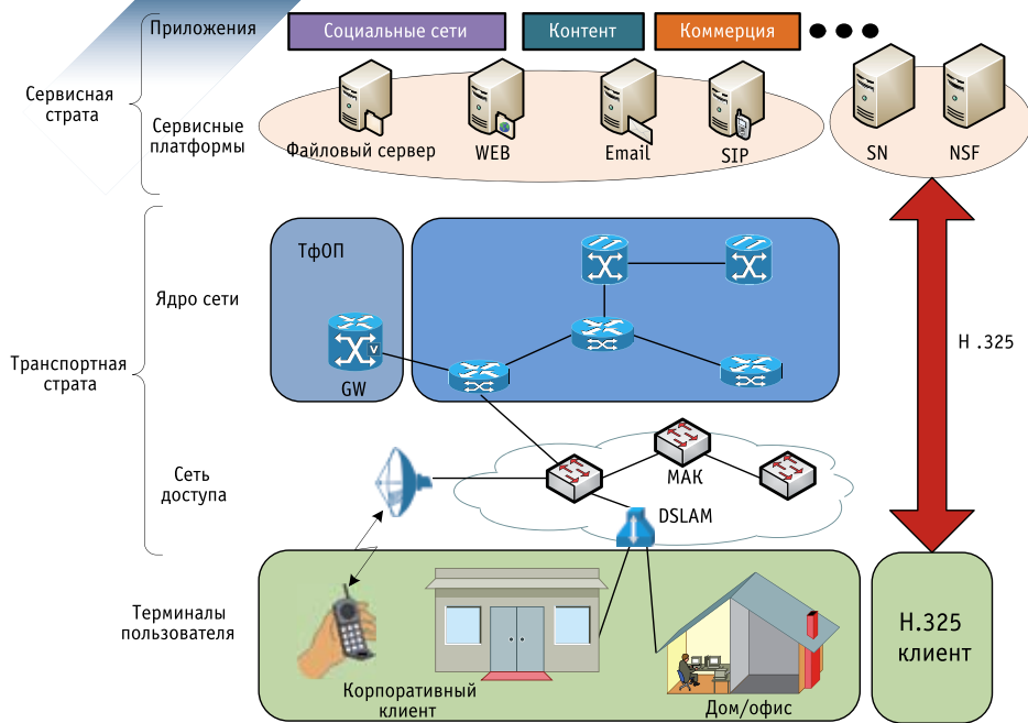
Рис. 3. NGN как транспорт для приложений AMS
