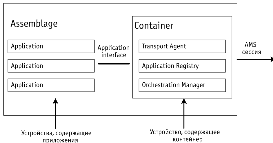
Рис. 2. AMS Assemblage
